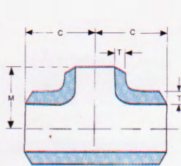
TEE
